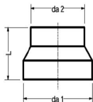
تبدیل هم مرکز پلی اتیلن مطابق استاندارد PE100/ISIRI14427
