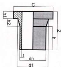
فلنج TYPE B پلی اتیلن مطابق استاندارد ۱۴۴۲۷/ISIRI/PE۱۰۰
