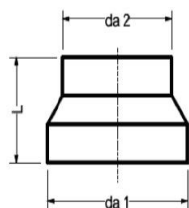
تبدیل هم مرکز پلی اتیلن مطابق استاندارد PE۱۰۰/ISIRI۱۴۴۷
