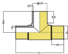
سه راهی پلی اتیلن مطابق استاندارد PE۱۰۰/ISIRI۱۴۴۲۷
