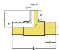
سه راهی پلی اتیلن مطابق استاندارد PE۱۰۰/ISIRI۱۴۴۲۷
